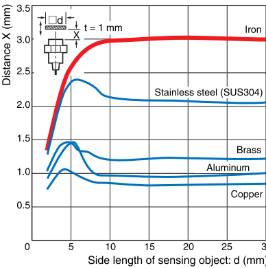
E2EH-X3□□
