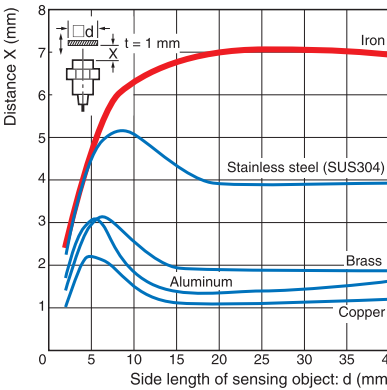
E2EH-X7□□
