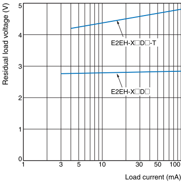
E2EH-X□□D□
