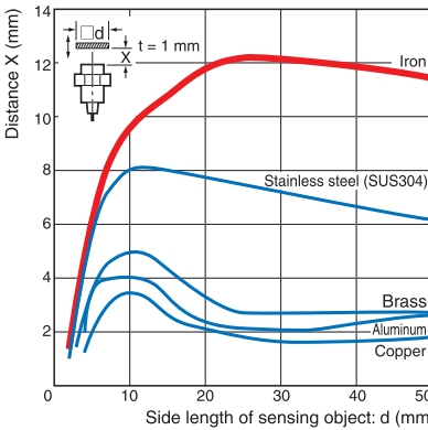
E2EH-X12□□
